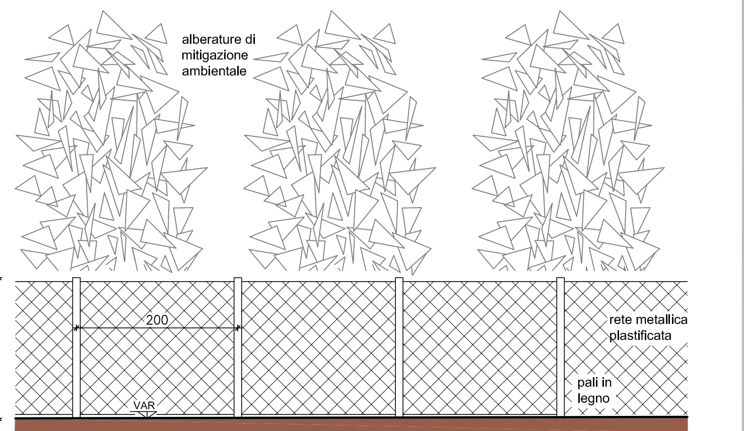
DETTAGLIO RECINZIONE - da 1 a 2 e da 4 a 1 scala 1:50
