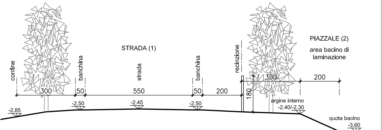
SEZIONE 1-1 scala 1:100
